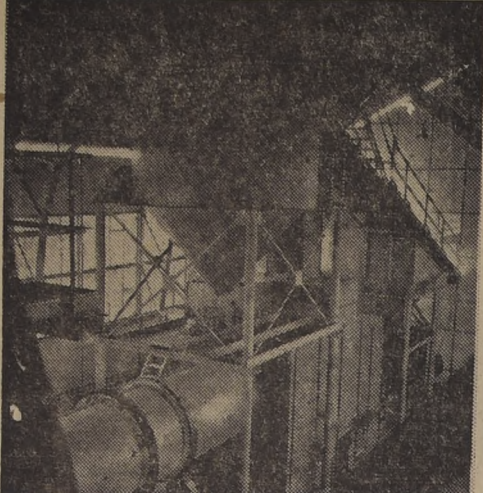
MECANIZACION DE FAENAS YESERAS. — El grabado da un aspecto del horno rotatorio de la moderna Fábrica de Yeso Romeral, organizada y dirigida por don Fernando Vargas Correa, que permitirá producir una cantidad prudencial de yeso para obras de construcciones. La mecanización de estas faenas es un paso en el avance industrial del país.
