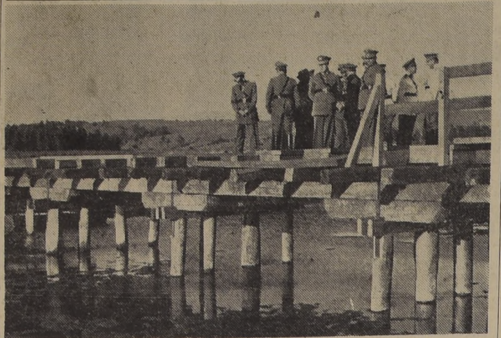
PUNTE Y CAMINO CONSTRUIDO POR MILITARES. — Este es el puente que sobre el estero de "Ventana" en Quintero, ha construido el Regimiento de Ingenieros N.º 2 de guarnición en Quilota, conjuntamente con el camino costero que permitirá mantener una constante comunicación en toda época del año. Actualmente, los vecinos tenían que dar vuelta por Puchuncaví, cuando se producían altas mareas. En el grabado el puente se inspecciona por el Ministro de Defensa Nacional, general señor Abdón Parra y jefes del ejército, durante la reciente visita que hizo a esa localidad.
