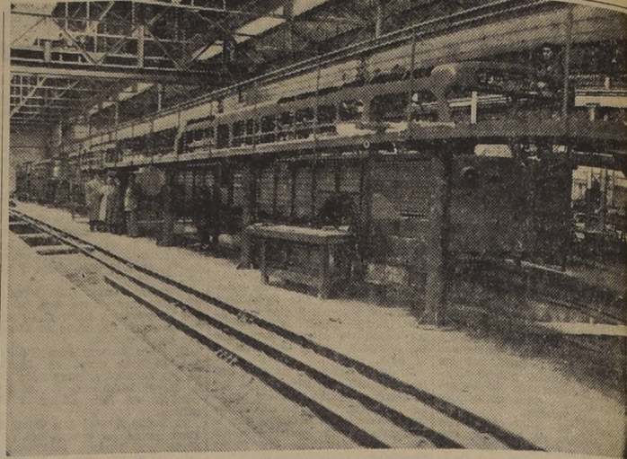
SOLUCION DEFINITIVA PARA LA LOCOMOCION COLECTIVA. — Aspecto interior de uno de los talleres mecánicos de la fábrica belga que está construyendo 100 trolleybuses marca "Vétra", destinados a nuestro país y que llegarán a puerto chileno a fines del mes de junio próximo, construidos a la Empresa Nacional de Transporte Colectivo del Estado. Se trata de moderna maquinaria, con capacidad de 48 personas cada una y que reúne toda clase de condiciones de confortabilidad. La construcción de estos aparatos está siendo supervisada en la fábrica por el ingeniero chileno Manuel Menéndez, de la Empresa Nacional de Supertránsito. Fácilmente se comprenderá que estos trolleybuses vendrán a satisfacer una sentida necesidad y que su importación forma parte del programa del Gobierno para solucionar definitivamente el problema de la locomoción colectiva.
