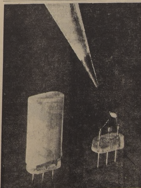
A LA IZQUIERDA, aspecto externo de un Transistor. A la derecha detalle interno, con sus tres alambres, placa y trozo de germanio, que son posteriormente recubiertos por una tapa de plástico. La punta del lápiz permite apreciar sus escasas dimensiones, no mayores que un grano de maíz.
