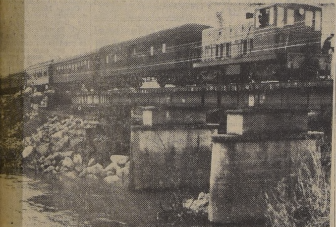
REANUDACION DE LAS COMUNICACIONES TERRESTRES.— Mañana quedará totalmente restablecido el servicio ferroviario al Sur del país, sin trasbordos, en razón de que han quedado totalmente arreglados los puentes destruidos por el último aluvión. En el grabado puede verse un convoy atravesando el puente de Pu. agán que fue destruido en una extensión de ochenta metros.
