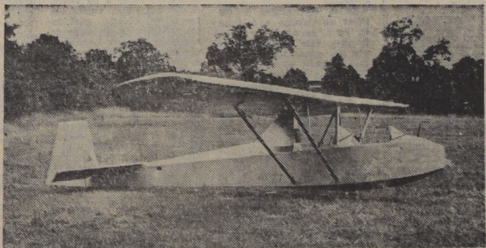
EL "SLINGSBY T. 31" Tandem Tutor, planeador de entrenamiento, de dos asientos. Tiene las mismas alas y cola que el "Tutor" original.
