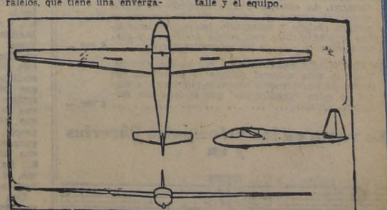
DISPOSICION general del "Crabpot 30", diseño original de Hugh Kendall, que ganó el concurso de diseño de la Asociación Británica de vuelos sin motor, en 1947. La versión modificada que se fabrica ahora, llamada "Miles M. 76", tiene alas, estabilizador en "V" y alerones plásticos.
