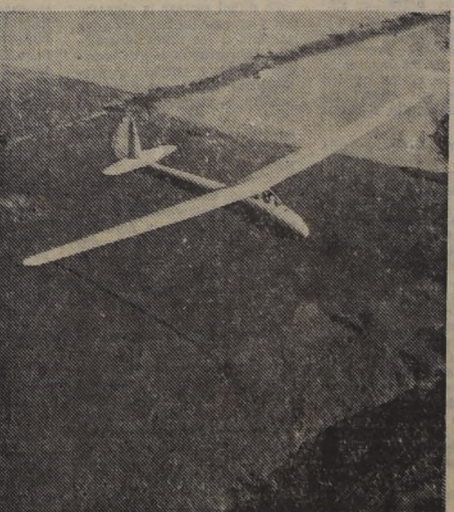
EL PLANEADOR "Sky", cuya performance se puso ampliamente de relieve en los Concursos Internacionales de Planeadores, celebrados en Madrid el año pasado. Este tipo de avión ganó 7 de los 14 puestos, incluyendo el primero
