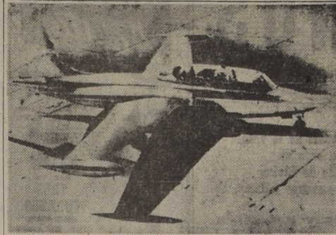
PARIS, junio 20.— El último aporte al equipo destinado a la compleja tarea de preparar pilotos para los cazas a reacción es el caso CM-170-E. El avión cuenta con un motor a reacción Fouga Special, con una cabina a presión para vuelos a gran altura y todos los elementos de combate, incluyendo ametralladoras, bombas, cohetes y dos tanques adicionales de gasolina en los extremos de las alas para las misiones a larga distancia. (Radiofoto UNITED PRESS)
