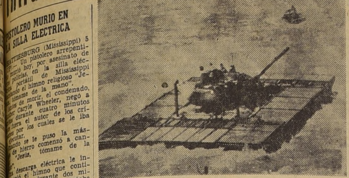
DETROIT.— Un tanque M-47 de 48 toneladas entra al Lago St. Clair durante pruebas de un nuevo aparato de flotación para esta clase de equipo que permite luchar mientras se "mecen" en las aguas. (RADIOFOTO UNITED PRESS).
