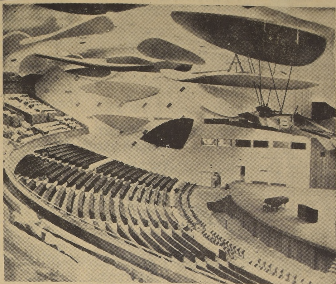
NOVEDAD ACUSTICA EN EL AUDITORIUM DE CARACAS.— Sala auditorium de la nueva Ciudad Universitaria de Caracas, donde se reúnen actualmente los delegados a la Décima Conferencia Interamericana. Sin ningún soporte interno para el techo de esta moderna sala, los espectadores, en cualquier punto de la sala pueden ver sin impedimentos lo que ocurre en el escenario. Además, el auditorium es con capacidad para 3.000 personas está equipado con un ingenioso sistema de paneles, que constituye una revolucionaria innovación en una teoría de acústica, pues la voz del orador en la tribuna es captada y desviada por estos paneles, transmitiéndola en igual volumen a todos los puntos de la sala.
