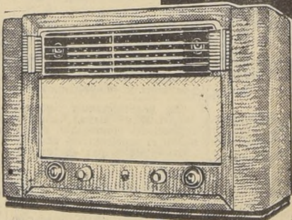
BSA-718-X Mueble enchapado en zebirano. Onda larga y corta ensanchada. 10 válvulas con 13 funciones. Parlante Ticonal de 10" con difusor. Enchufes para Pick-up y para parlante adicional. Ojo mágico
