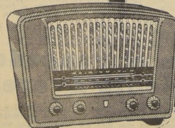
BSA-326-U Gabinete de madera. Dial y rejilla plásticos. Ondas larga y corta. 5 válvulas con 8 funciones. Corriente universal. Parlante Ticonal de 7" Enchufe para Pick-up
