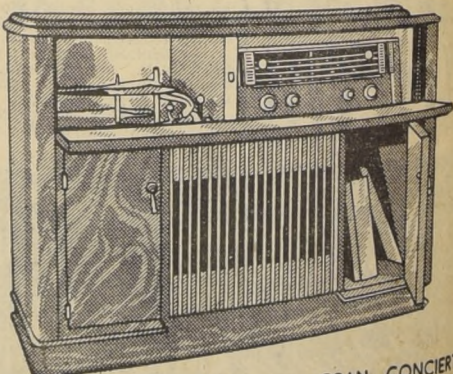
FSA-819-A GRAN CONCIERTO Mueble enchapado en caoba. Onda larga y corta ensanchada. 10 válvulas con 13 funciones. Parlante Ticonal de 12" con difusor. Ojo mágico. Pick-up con cambiador automatico de 3 velocidades
