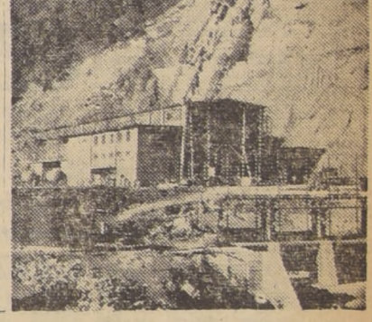
EN "LOS CIPRESSES". — Tres aspectos de la intensa actividad que desarrollan los hombres y las máquinas para terminar rápidamente la nueva central hidroeléctrica de LOS CIPRESSES, en la provincia de Talca. Arriba, vemos una de las modernísimas "torres dosificadoras de concreto", que han sido elementos determinantes en la velocidad de las faenas. En el ángulo derecho, los obreros que construyen la "cinturón de equilibrio", enclavada en plena roca, 358 metros más arriba de la Casa de Máquinas, obra de ingeniería que será única en Chile y que permitirá regular el paso de agua a las turbinas. almacenándose pasajera y momentáneamente. A la derecha, podemos apreciar, en vista panorámica, la Casa de Máquinas, con la tubería aún inconclusa y sus túneles, de desagüe. Aquí se han instalado las tres enormes turbinas que generarán los 92.500 KW que producirá esta planta.
