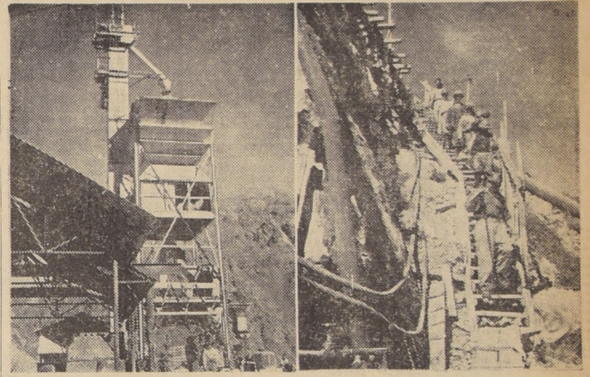
EN "LOS CIPRESSES". — Tres aspectos de la intensa actividad que desarrollan los hombres y las máquinas para terminar rápidamente la nueva central hidroeléctrica de LOS CIPRESSES, en la provincia de Talca. Arriba, vemos una de las modernísimas "torres dosificadoras de concreto", que han sido elementos determinantes en la velocidad de las faenas. En el ángulo derecho, los obreros que construyen la "cinturón de equilibrio", enclavada en plena roca, 358 metros más arriba de la Casa de Máquinas, obra de ingeniería que será única en Chile y que permitirá regular el paso de agua a las turbinas. almacenándose pasajera y momentáneamente. A la derecha, podemos apreciar, en vista panorámica, la Casa de Máquinas, con la tubería aún inconclusa y sus túneles, de desagüe. Aquí se han instalado las tres enormes turbinas que generarán los 92.500 KW que producirá esta planta.
