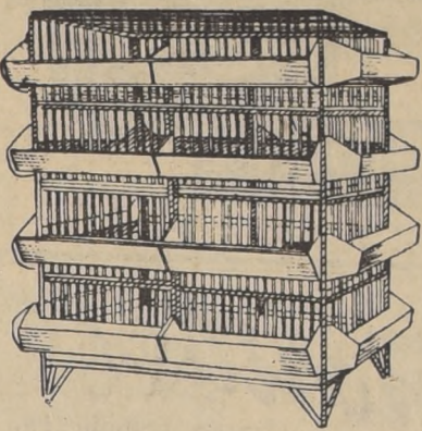
BATERIA DE RECRÍA, TIPO BUCKEYE, PARA 400 POLLOS HASTA LAS 12 SEMANAS
