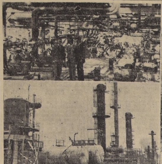
LA REFINERIA DE CONCÓN.—Tres interesantes aspectos de la Refinería de Petróleo de Concón, que en el mes de agosto próximo iniciará sus actividades, marcando un paso de importancia hacia nuestra independencia industrial y económica.— Atriba, a la derecha, don Manuel Ossa Saint Marie, pionero de la industria del petróleo en Chile
