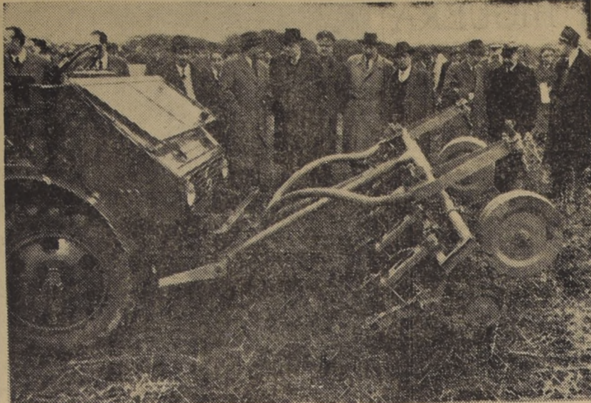
EL "UNIMOG" EN ACCION. — El Presidente de la República, Ministros de Estado y altos funcionarios de la CORFO presencian al tractor UNIMOG en pleno trabajo, accionando una cultivadora mediante dispositivos hidráulicos. Fue realmente una buena prueba de eficiencia, dijeron, los asistentes al campo militar de Peñalolén.
