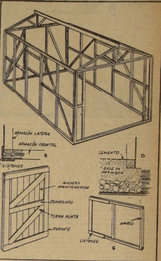
Garage desarmable de 4,90 metros por 3 metros.
