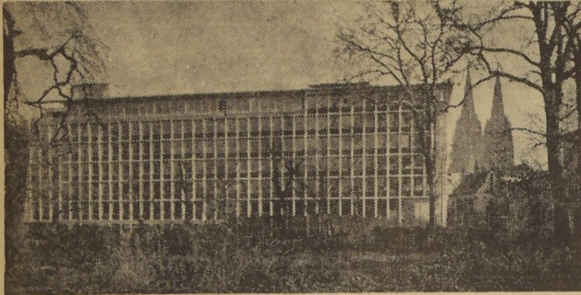
Arquitectos: Wilhelm Riphahn y Paul Doetsch. Sociedad Constructora CONCORDIA. Edificio de departamentos en Kilm, Alemania. La característica primordial de este bello edificio, es la angostura de sus costados, en la que juega una importancia capital la construcción de plástico, vidrio y metal, la que a pesar de su fina
