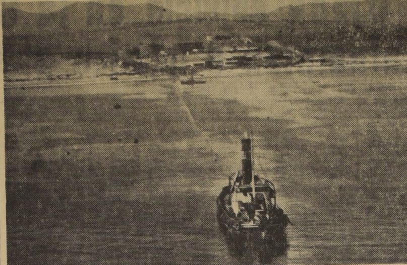
COLOCAN TUBERIA SUBMARINA.— Vista aérea tomada desde el momento en que el remolcador "Kangaroo" termina de amarrar el extremo de la cañería submarina de 1.480 metros de longitud, que servirá para descargar en el fondo del mar el petróleo que irigan desde Manantiales los barcos-cisternas. — (TAGLE, corresponsal).
