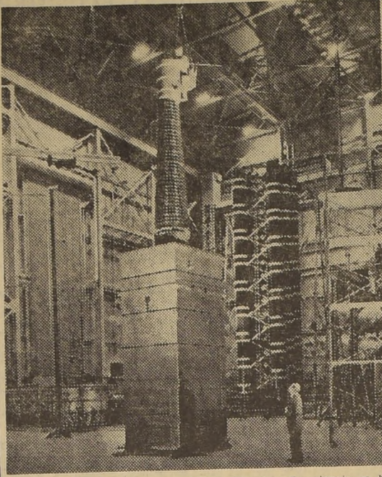
PITTSFIELD, Massachusetts, (Globe Press). — La ciencia se ha visto sorprendida frente a la construcción de uno de los más grandes transformadores que se han producido en los Estados Unidos. La General Electric entregó este aparato, cuyo potencial está clasificado como el mayor del mundo. Tiene una altura de 10,58 metros, pesa 50,000 libras y tiene un contenido de 50 millas de alambre de cobre, con más de 3,000 libras destinadas a su aislamiento eléctrico. Permite la reducción del voltaje y los estudios que a través de él se realizan, revisan de una vital importancia para la industria eléctrica en los Estados Unidos. El grabado lo muestra mientras un especialista, montado en una silla mecánica a una altura de tres pisos, está haciendo una revisión, bajo la supervigilancia de otro experto. Su producción, que podría ser vital en el futuro, está siendo contemplada, como de trascendente importancia en el ramo. — (Foto Globe Press).
