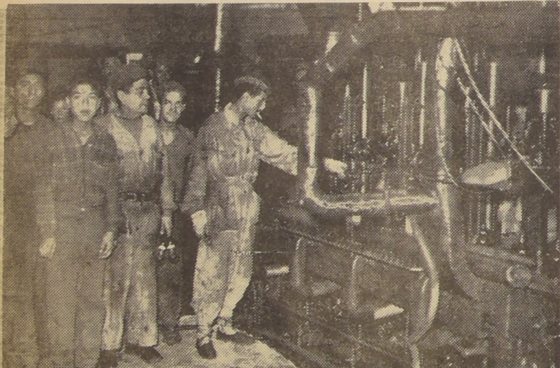
MAQUINARIAS DEL PROGRESO. —Mostrando su enorme estructura, esta máquina destinada a la fabricación de artículos de vidrios, es un mudo exponente del progreso de la industria nacional.
