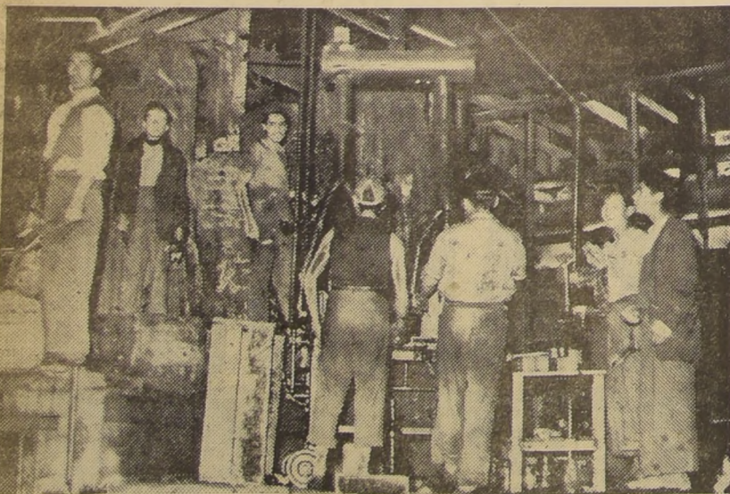
DELICADA LABOR. —Obreros chilenos, al servicio de una firma chilena, son los trabajadores de las Cristalerías de Chile S. A. Dos de ellos aparecen en delicadas labores, junto a las válvulas de seguridad de uno de los hornos.
