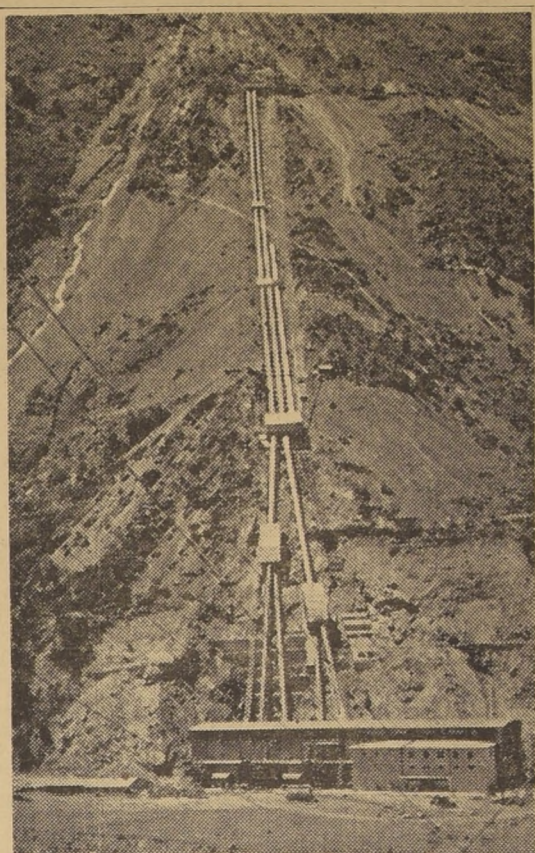
FUENTE DE PROGRESO. — Así, como la muestra el grabado, es hidroeléctrica de Los Cipreses, a 90 kilómetros de Talca, en un bello rincón de la cordillera. Cada uno de los tubos que se observa en el grabado, está constituido por el ensamble de sectores de seis metros, con un espesor de una pulgada, que se van subiendo por funicular. La tubería, por sus complejas especificaciones técnicas, no pudo ser construida en Chile, y se encargó a la firma Mannesman, de Alemania.
