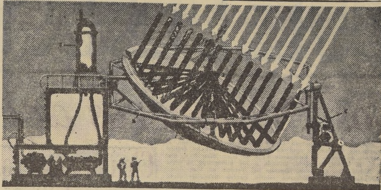
MOTOR SOLAR ABBOT — El espejo parabólico (A), montado en balancines (B), movido por relojería (C), sigue al Sol. Los rayos solares (1) enfocados al tubo calorífico (2), convierten agua en vapor dentro de la caldera (3). El vapor mueve a la turbina (4) y mueve a la dinamo (5). El exceso de calor se acumula en la cámara (6).
