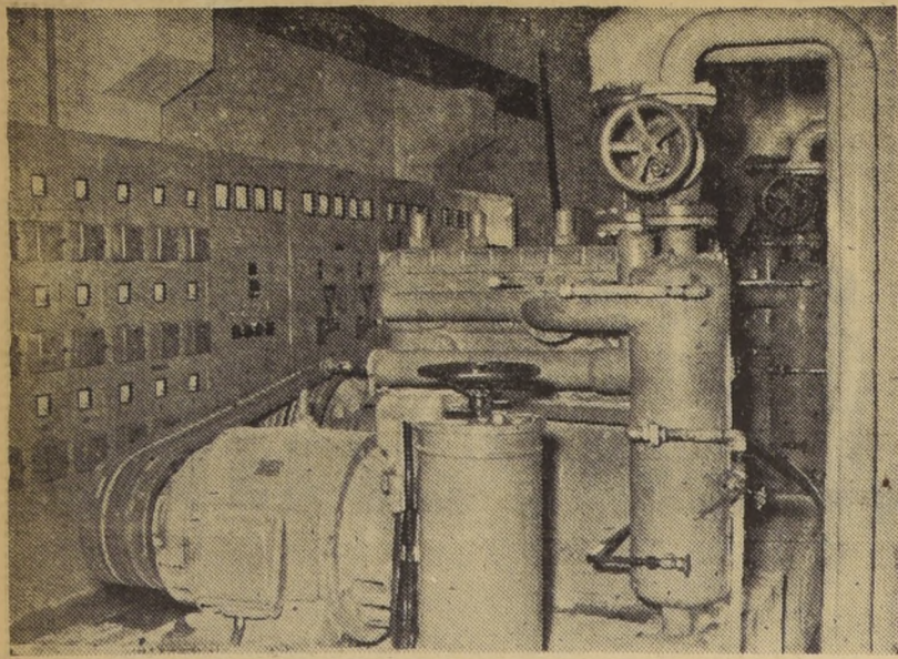
SALA DE MAQUINAS. — El grabado muestra un aspecto de la Sala de Máquinas del Frigorífico de Talcahuano, las cuales son capaces de producir 640 mil calorías-hora, o sea, 210 mil toneladas de refrigeración. La maquinaria comprende cuatro compresores verticales, cuatro condensadores, dieciocho evaporadores, una subestación eléctrica y un sistema de control automático de temperatura.
