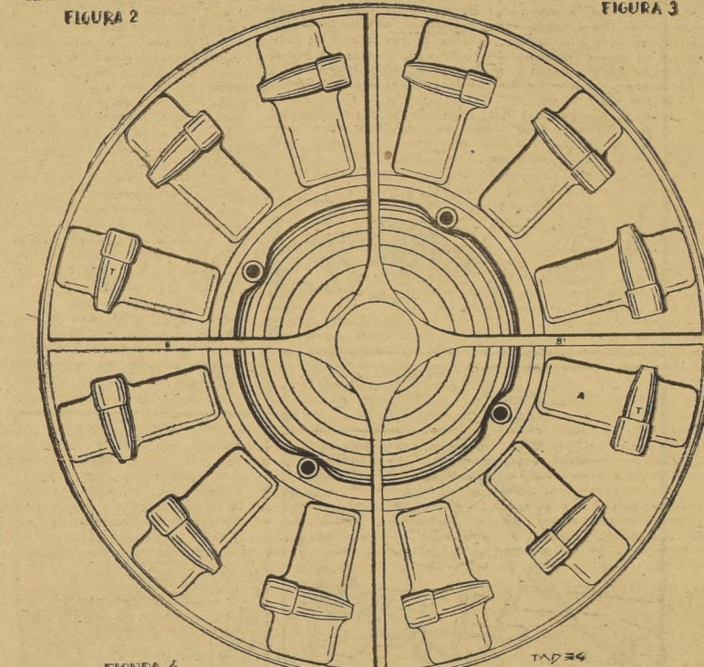
Figura 1.— CORTE DEL DISCO.— A) Aletas del Turbo-impulsor. A-c) Aletas compensadoras de estabilidad. B) Brazos interiores huecos. B-1) Brazos exteriores macizos. C) Conductores de gases. G) Tubos de gases para los turbo-reactores. G-1) Giróscopos. M) Motores de los giróscopos. O) Depósitos de oxígeno. P) Piso de la cabina. T) Toberas de turbo-reacción. T-1) Tablero de distribución. V) Varilla de aceleración, cambio de ángulo de las aletas y chispa. X) Baterías. El generador de corriente continua que va accionado por el eje del motor de impulsión va detrás del tablero de distribución. Figura 2.— EN VUELO DE COHETE. Figura 3.— EN VUELO HORIZONTAL (Vuelo de Helicóptero). Figura 4.— VISTO POR ENCIMA.
