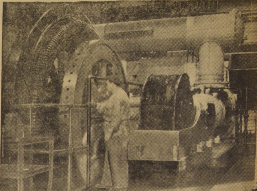
PODEROSAS MAQUINARIAS. — En el interior de la mina se han instalado maquinarias de gran volumen. La subestación, a 500 metros de profundidad horizontal y 500 de profundidad vertical, proporciona abundante iluminación y energía para mover todo el sistema interior de la mina y las instalaciones de aire acondicionado.
