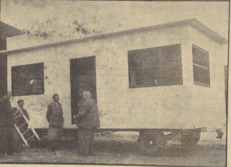
Una casa prefabricada resistente a terremotos ha sido recientemente construida en Islettes y trasladada por tierra, para ser presentada en la Feria de París. Está hecha de bloques de concreto colocados sobre marcos de madera de un metro por cincuenta centímetros. El interior está tapizado en madera. La casa consta de dos piezas: una sala y un dormitorio. Su precio debe ser de 500.000 francos aproximadamente. Durante la exhibición en la Feria de París, estará sometida a movimientos tan intensos como los de un verdadero fuerte temblor. (Foto Intercontinental)
