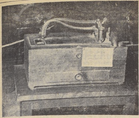
Primera máquina de coser introducida a Chile, fabricada por Howe, y traída por la señora Caleta Larrain de Dávila. — (Museo Histórico Nacional)
