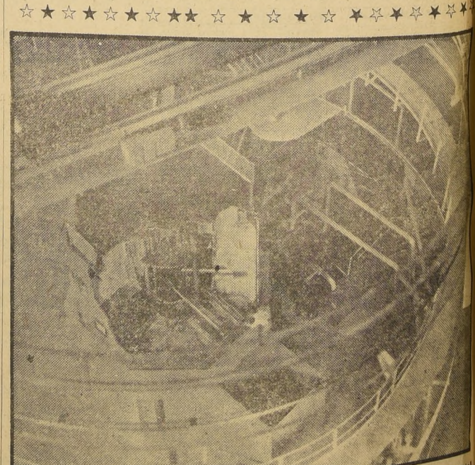
3 PORCION CORRESPONDIENTE al reactor, propiamente tal, del Reactor Experimental de Agua Hirviendo del Laboratorio de Argonne. La cámara de presión, que se presenta en corte, contiene elementos combustibles productores de uranio, con varillas de control que absorben los neutrones. El vapor generado en la cámara de presión es enviado por un separador a la turbina que se ve en la parte superior.
