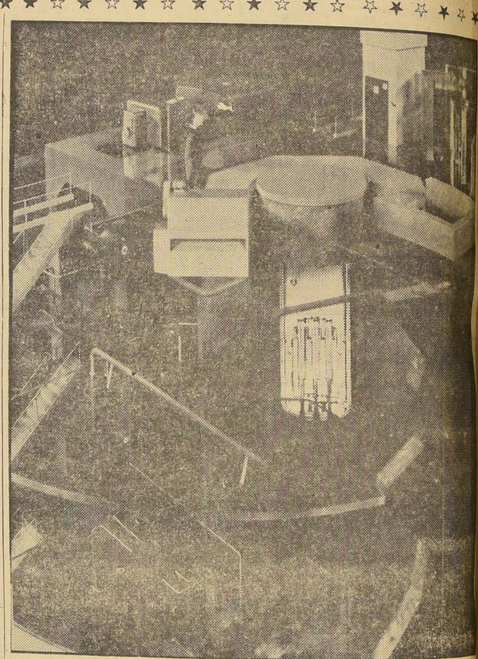
2 HE AQUI un corte que revela íntimamente del reactor de investigación, perteneciente al Laboratorio Nacional de Argonne, EE. UU. Se trata de un reactor de agua pesada, moderado y refrigerado, construido en 1953. La sección en corte muestra el conjunto de elementos combustibles productores de uranio, y las instalaciones experimentales.
