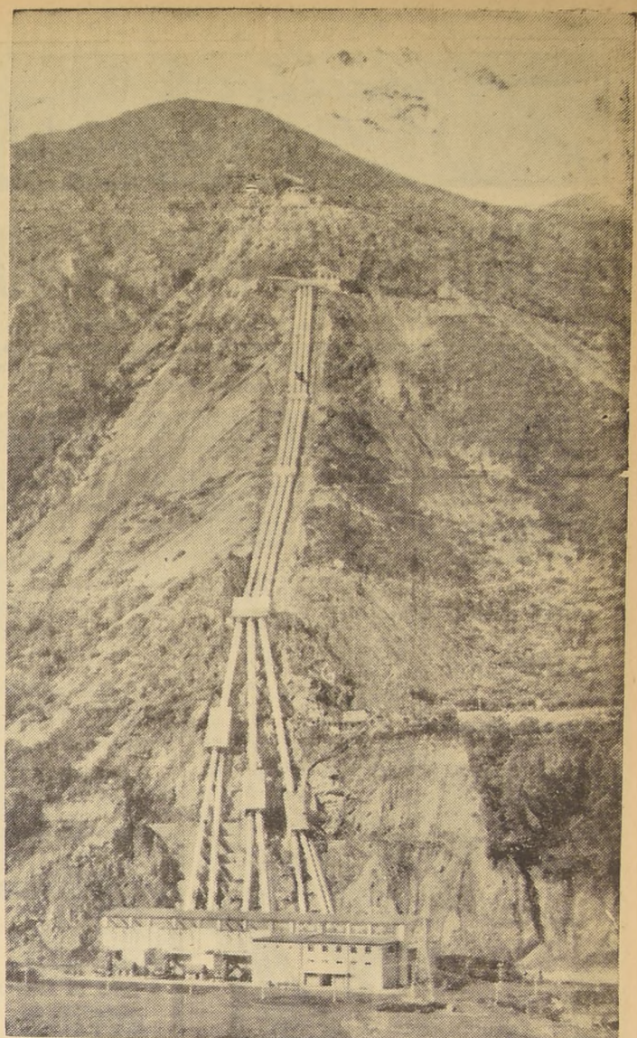
VISTA GENERAL DE LA CASA DE MAQUINAS Y DE LAS TUBERIAS
