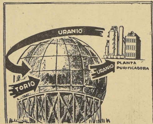
Dentro del "reactor de incubación" el metal torio entra a una área que rodea el centro de este gigante aparato. Los neutrones del núcleo transmiten al torio en una forma de uranio fisionable (U-233). El vapor canalizado desde el reactor genera electricidad. El uranio del reactor es purificado en una planta química. Después sirve de combustible para aviones, trenes o buques atómicos. Una pequeña parte de él sigue alimentando al reactor incubador.
