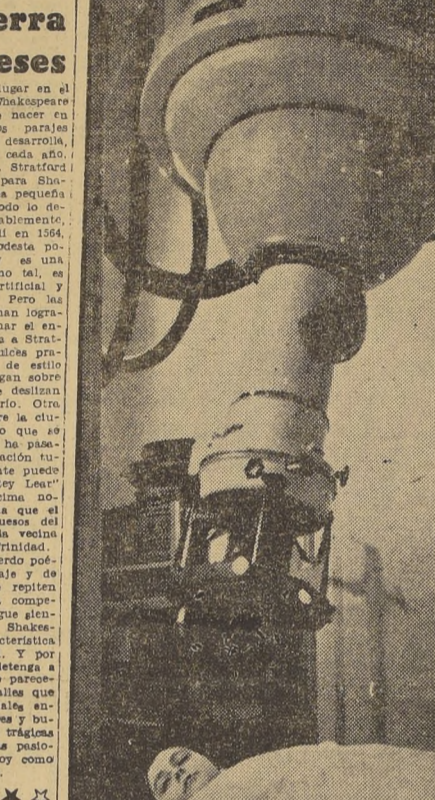
HE AQUÍ una de las más modernas máquinas, destinadas al tratamiento del cáncer por irradiación. Trata de una máquina de Rayos X de un millón de voltios. Según los dos mil sabios, recién reunidos en la Conferencia Atómica Mundial de Ginebra (Suiza), el tratamiento del cáncer mediante los isótopos radioactivos, registra éxitos verdaderamente milagrosos.
