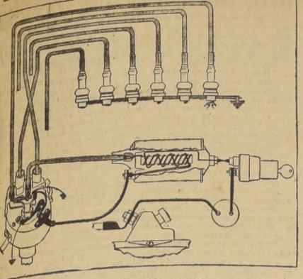
Estos son los circuitos del encendido. Las líneas negras pesadas indican el circuito primario; interruptor de arranque al amperímetro; el interruptor de encendido; al arrollado primario de la bobina; al condensador y el circuito secundario; a tierra. Las líneas sombreadas indican la tapa del distribuidor; al arrollado de la bobina a la tapa del distribuidor; al rotor; a los segmentos de la tapa; a las bujías, y a tierra.
