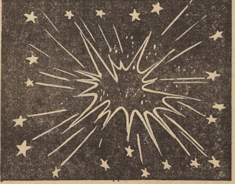
Una explosión estelar que según astrónomos chinos acaeció en 1054, antes de Cristo, dejó una nube de gas conocida por la Nebulosa del Cangrejo, que actualmente expandiéndose a 1.100 Kms. por segundo. Su diámetro actual es de 34 años luz.
