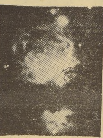
La promigiosa Nebula de Orion. Nuevos astros nacen continuamente en el Universo.
