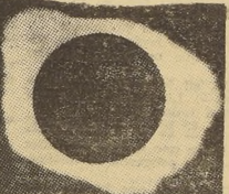
La Corona Solar: un halo de fuego venido de otras estrellas.
