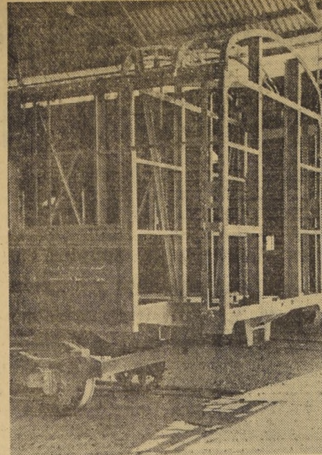
Este es uno de los carros que Socometal entregará próximamente a Ferrocarriles del Estado, y que reemplazarán a los de madera actualmente en circulación. La terminación es completamente metálica, con el acero chileno, como puede apreciarse en la fotografía de la parte de atrás del carro. Obvio es decir la resistencia que tiene para cualquier emergencia. Actualmente la entrega se encuentra paralizada por carecer la industria de divisas para traer ciertos elementos indispensables del extranjero. Pero, solucionada esta dificultad y contando con todos los medios a su alcance, Ferrocarriles podría, en el plazo de un año y medio, reemplazar todo el material rodante de frágil madera.
