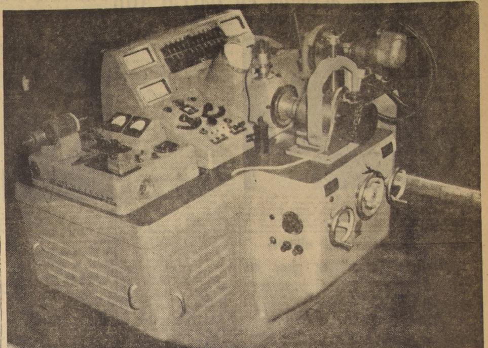
Este moderno banco de prueba para motores permite que cada máquina ajustada en los talleres de la Agrotecnica S. A. C. I. sea revisada hasta en sus más mínimos detalles, de manera que el motor tenga las características de funcionamiento de un motor recién salido de fábrica, completamente nuevo.
