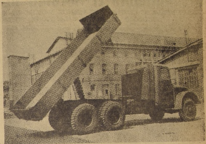
Camión de volquete TATRA 111-S, con dispositivo volador al aceite, para los tres lados. Su motor es de 12 cilindros en V, y desarrolla 180 H. P. a 1.800 r. p. m., con una cilindrada de 14.825 cm 3 . Funciona a gasoil y es refrigerado por aire.
