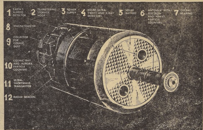
Vista esquemática del satélite "MOUSE", con sus múltiples y complicados instrumentos: 1) detector albedo terrestre; 2) telémetro; 3) batería; 4) detectores de Rayos X y ultravioleta; 5) acumulador; 6) antena solar; 7) rodamiento universal; 8) magnetómetro; 9) colector de polvo cósmico; 10) contadores de rayos cósmicos; 11) transmisor onda ultracorta; y 12) emisor de radar.
