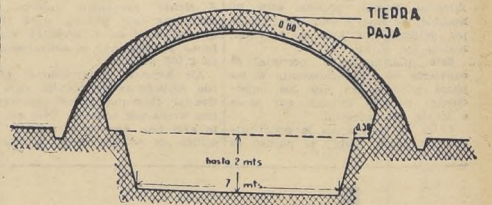
CORTE LONGITUDINAL DE UN SILO ZANJA
