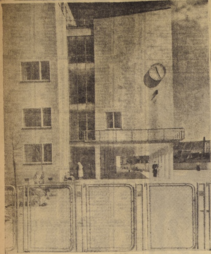
Escuela para muchachas, en Norrmalm, Estocolmo, por N. Ahrbom y H. Zmdahl. Este es un buen ejemplo de la arquitectura sueca del decenio 1930 a 1940.
