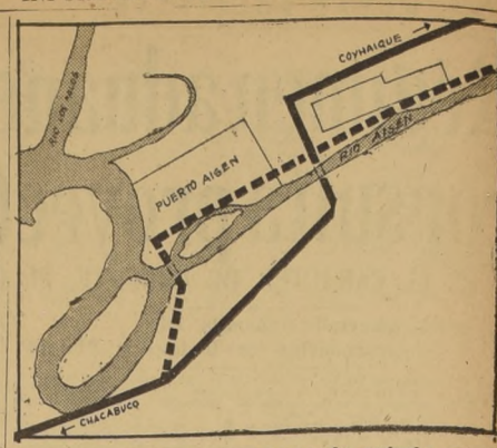
En el croquis pueden apreciarse los trazados profundos para el puente sobre el río Aisén: la línea negra, del Ministerio de Obras Públicas, y la cordada, de los vecinos de la zona.
