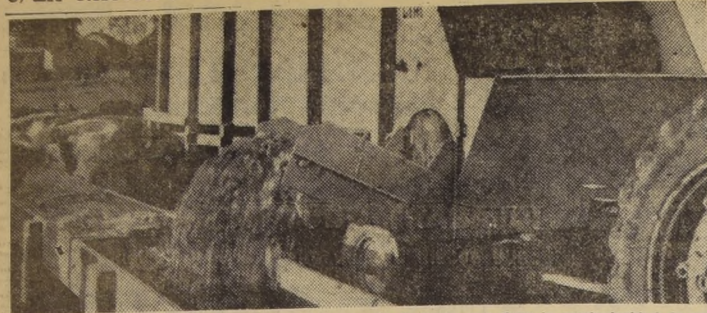
En el grabado, un trailer con box para el transporte de pasto, que tiene la particularidad de expulsar su contenido por una tolva directamente a las canoas de alimentación del ganado. El desplazamiento del box se realiza mecánicamente mediante un sencillo sistema de engranajes. Este equipo está especialmente indicado para facilitar la adecuada alimentación del ganado por "soiling". Su diseño pertenece a la firma "Gehl", y está siendo muy difundido en los Estados Unidos, por su facilidad de operación y el ahorro de mano de obra que representa.
