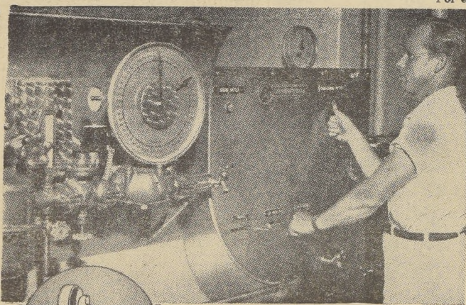
Activado por botón, el tablero de control dosifica las cantidades apropiadas de azúcar, fermentos y otros aditivos para la máquina elaboradora de pan.
