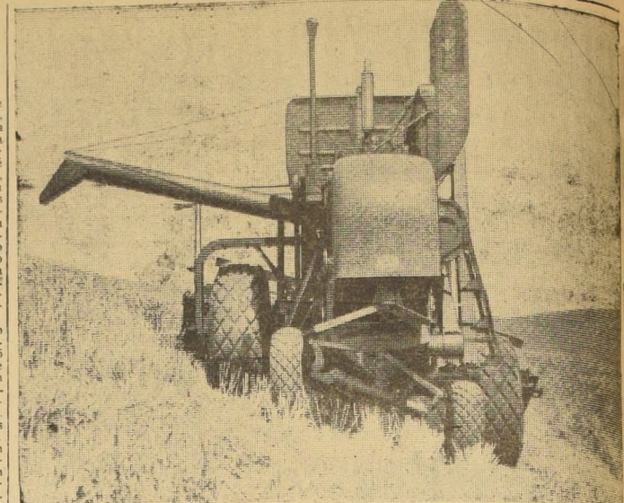
En el grabado una sembradora combinada, especialmente adaptada para los trabajos de cosechar en suelos ondulados. La movilidad de sus ruedas permite a esta máquina cosechar sin dificultad en cerros sembrados de cereales. Con este nuevo tipo de sembradora, el problema de la cosecha en esta clase de terrenos queda solucionado. La maquinaria del grabado es importante para el país ya que gran parte de los suelos de los cereales son de relieve.
