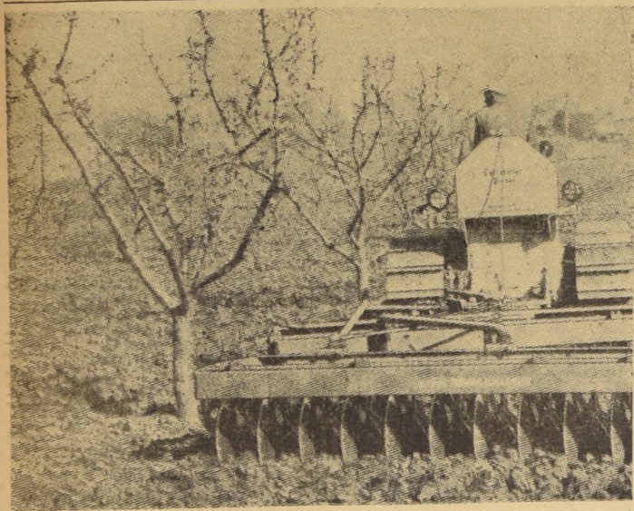
En el grabado se muestra el trabajo del suelo de un huerto frutal. Obsérvese el estado de movimiento del suelo, que es laborado mediante una rastra de discos OFF-SET, la cual permite dar una raja de tipo mediano, muy indicada para las arboledas.
