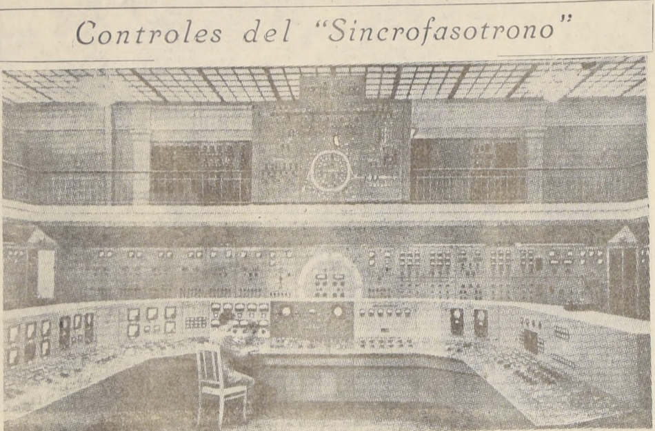
Una vista panorámica de la gran sala de mando, desde donde se controla el funcionamiento del gigantesco "sincrofásotrono", construido por los sabios soviéticos para el Instituto Unificado de Investigaciones Nucleares de la URSS.
