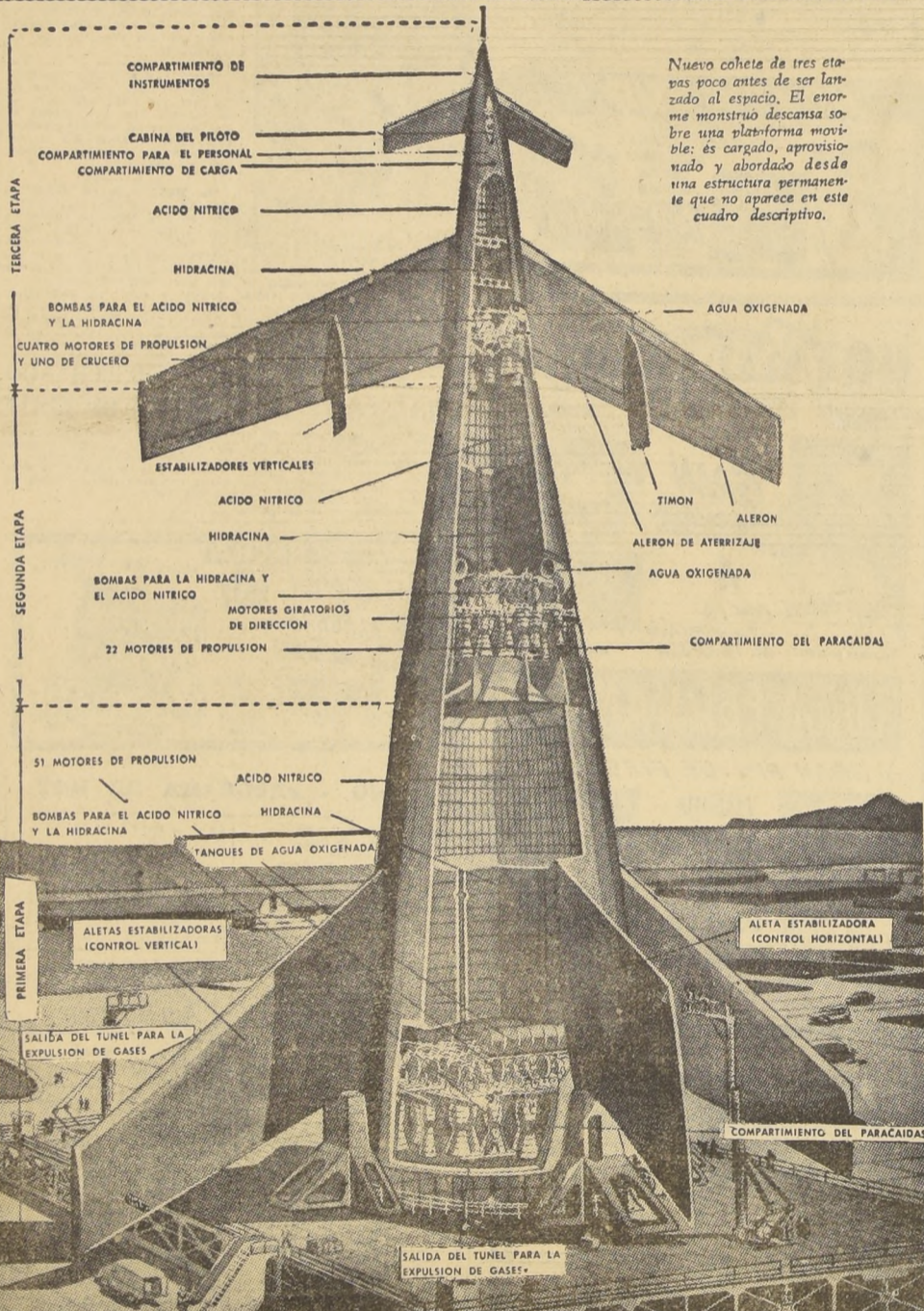
LA NAVE ESPACIAL.— La nave del espacio será también un cohete de tres secciones, iguales que los que dispararon los Sputniks I y II, pero en su cúspide, en vez de llevar un satélite artificial, llevará un avión, que volará en la última etapa, perfectamente manejable por control remoto. Si los pilotos, por
