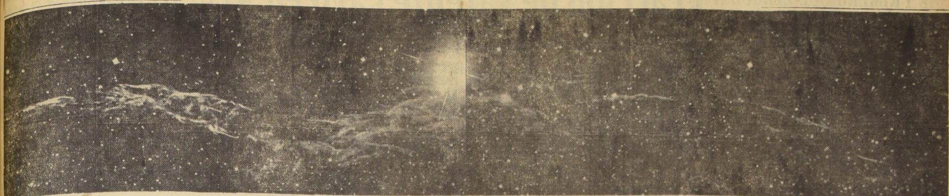
EL CISNE, una nebulosa muerta hace ya millones de años. Aparece en el grabado grabada con una exposición de 100 horas. Esta imagen a la vista de los terrestres parece una realidad presente, pero es sólo visión del pasado, por que estas nebulosas han muerto al perder su luz propia hace millones de años. Para explicar este fenómeno habría que invertir el proceso: si en este momento, desde Cisne, alguien enfocara un poderoso telescopio hacia la Tierra, la visión que esta presentaría, correspondería al periodo de Cristo o el incendio de Roma, pues estaría mirándonos desde un lugar situado a dos mil años luz. Un año luz es la distancia recorrida por un haz luminoso en 365 días a la velocidad de 300 mil kilómetros por segundo. La Constelación del Cisne, en la Vía Láctea, fue descubierta por Ptolomeo, quien le dio tal nombre y en ella se encuentra la estrella 61, la primera en que se descubrió movimiento propio. Ahora el hombre se encuentra en el amanecer de una nueva Era en el estudio de los espacios siderales a través de los satélites artificiales y los cohetes teleguiados.
