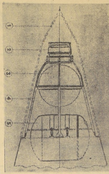
MOSCU.— Este es un diagrama del Sputnik II, como se ha publicado en el diario oficial soviético "Pravda", el 13 del presente. Según la leyenda que acompaña el dibujo, los números representan lo siguiente: 1) Como protector arrojado al espacio después que el Sputnik entra a su órbita; 2) Aparato para investigar los rayos ultravioletas y rayos X de la radiación solar; 3) Depósito con aparato transmisor de radio; 4) Marco sobre el cual están fijados los aparatos; y 5) Cabina de la perrita Laika.— (Radiotelegramas de la UNIÓN PRESS.)
