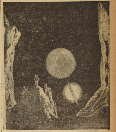
El sistema de estrellas dobles Beta, de la Constelación del Cisne, visto desde uno de sus planetas. El estudio de las estrellas dobles fue posible gracias a las leyes de Kepler, ya que una estrella gira en torno de la otra de la misma manera que la Tierra alrededor del Sol. Las mismas leyes permiten deducir también la existencia de planetas en algunos casos, aunque los telescopios no sean capaces de confirmar, mediante la observación, la exactitud de los cálculos. En el grabado, sobre la roca central, cuatro soldados de las naves interestelares del futuro, montan guardia.
