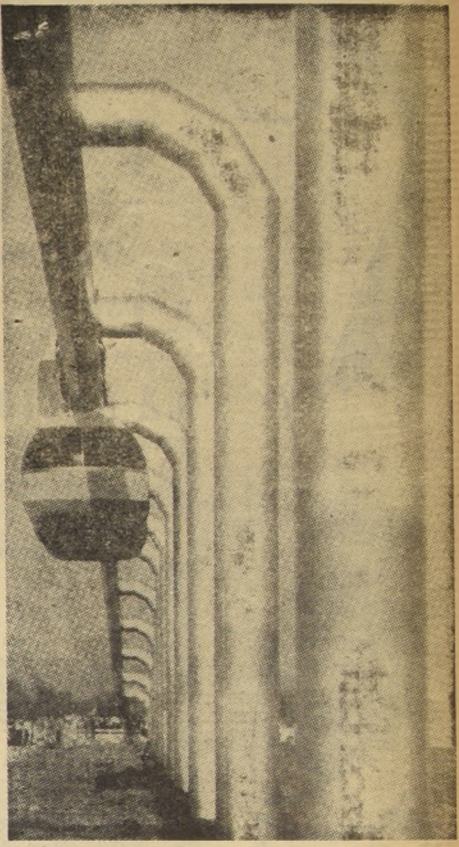
Se exhibió, no hace mucho, en Houston, Texas, el primer tren monorriel aéreo norteamericano. Ante las muchedumbres que se turnaban para subir a él, un vagón impulsado por motor de gasolina iba y venía por un trayecto de casi 300 m. de longitud (abajo). Los constructores de este vehículo, la Monorail Inc., de Houston, dicen que su fabricación resulta más económica que la de los demás ferrocarriles urbanos y esperan que el sistema interese a las ciudades con problemas de tránsito.
