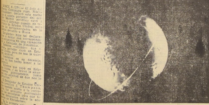
En el grabado, la ruta que sigue el Sputnik II a través del espacio, a 1.500 kilómetros sobre la superficie de la Tierra. La fotografía corresponde a un documento soviético filmado en Rusia con motivo del lanzamiento del segundo satélite artificial ruso.
