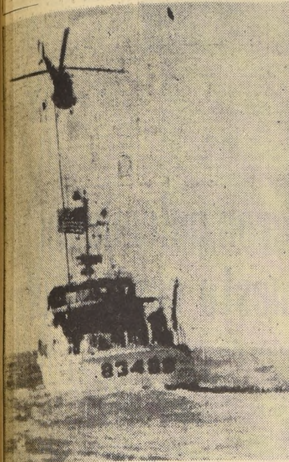
PETERSBURG (Florida).— Un helicóptero Sikorsky, de la Guardia Costera de los Estados Unidos, con todo éxito remolca un barco patrulla de 78 toneladas, en una prueba realizada aquí el día 10. El helicóptero remolcó la embarcación, de 83 pies de largo, en una distancia de 10 millas.— (Radiofoto UNITED PRESS.)
