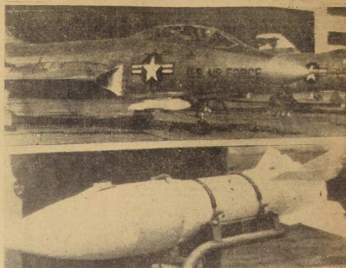
NEUVA YORK.— La McDonnell Aircraft Co. dio a conocer el 15 del presente su último modelo de avión de combate. Dicha máquina, accionada a retroimpulso, transporta en la parte inferior un proyectil cohete Woodcock (que aparece en la foto de abajo), el cual se despiiza a una velocidad de 1.900 kilómetros por hora.
